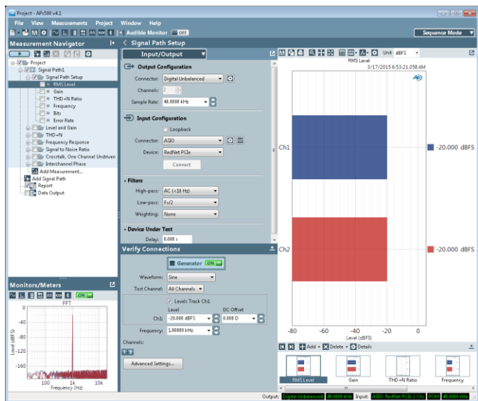
図 17. APx による RedNet 3 SPDIF 入力から Dante Tx シグナルパスの測定画面
